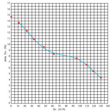
Fan efficiency characteristic Lüfterleistungskennlinie Caractéristique du débit de ventilateur
